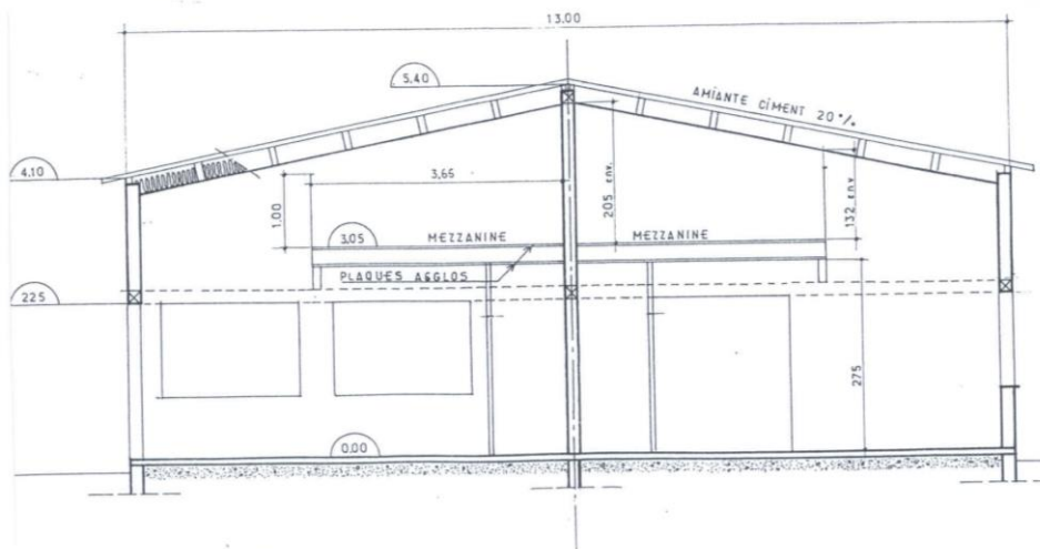
COUPE XX
